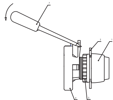
Rys. G Sposób demontażu napędu z pulpitu
