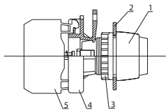
Rys. A Człony funkcjonalne przycisków i lampek
