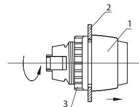
Rys. G Sposób demontażu napędu z pulpitu
