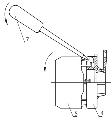
Rys. F Sposób demontażu korpusu pośredniego
